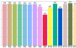
CRI: 92.4 (R1-R8)
